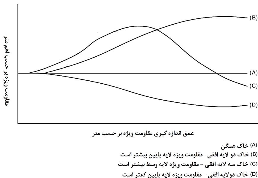
شکل ۳-۲ - منحنی تغییرات مقاومت ویژه بر حسب فاصله الکترودهای تست [۶]
