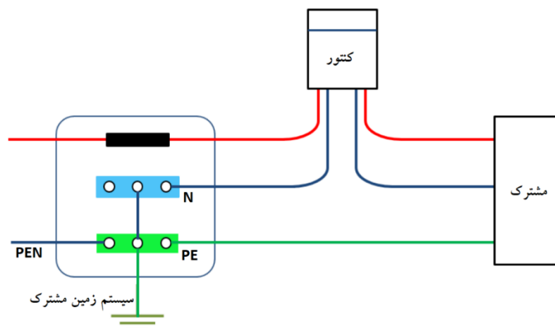
شکل ۴-۲۰- نحوه تفکیک PEN به دو شینه نول و PE
