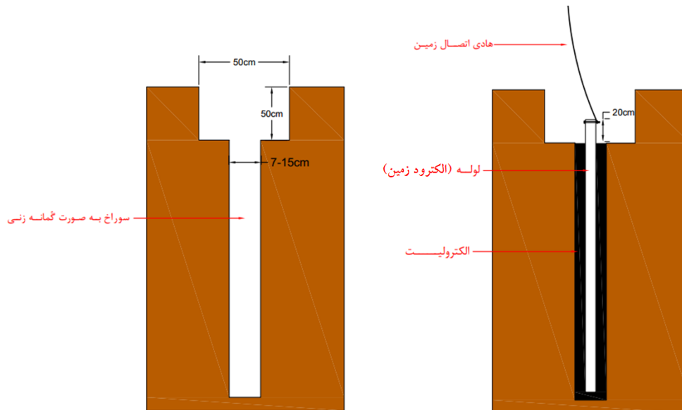
شکل ۵-۶- نحوه اجرای الکترود قائم با استفاده از ماشین آلات حفاری
