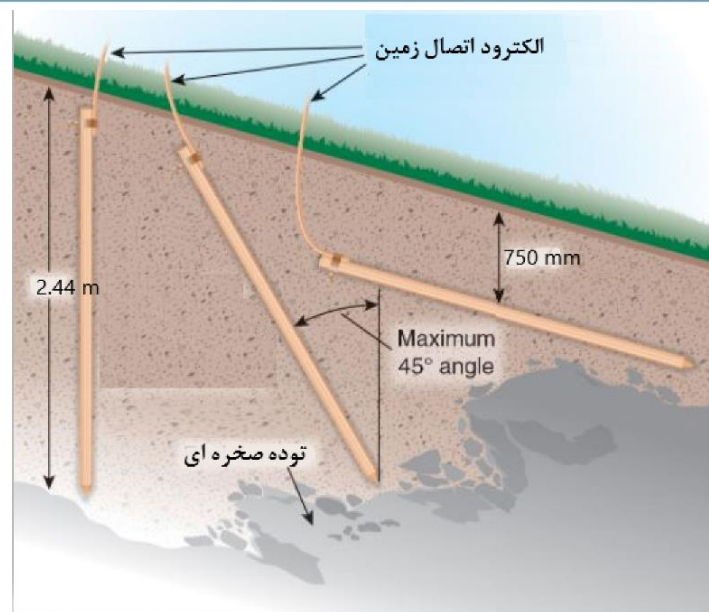
شکل ۵-۵- شکل های مجاز اجرای الکترودهای میله‌ای
