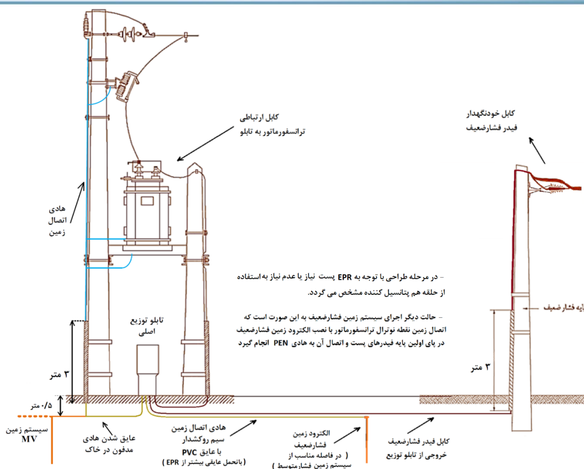
شکل ۴-۲- اتصال زمین سمت فشار ضعیف و فشار متوسط پست هوایی
