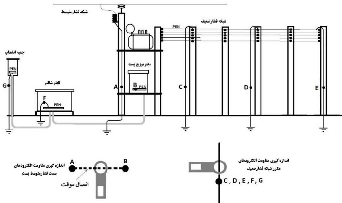
شکل ۳-۶- اندازه‌گیری مقاومت سیستم زمین به روش تزریق جریان کلمپی
