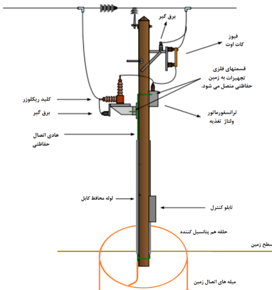
شکل ۴-۹- نحوه زمین کردن تجهیزات قطع کننده فشار متوسط هوایی دارای تابلو کنترل در ارتفاع پایین ۱
