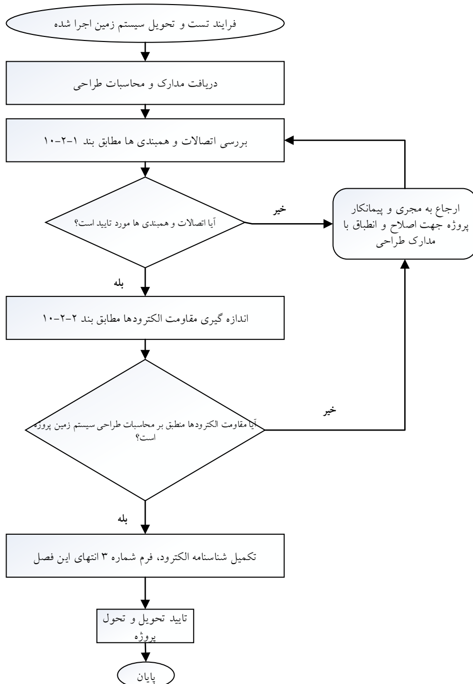
شکل ۶-۱- فرایند تحویل و تحول سیستم زمین اجرا شده
