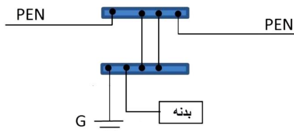
شکل ۴-۳- اتصال زمین تجهیزات در شبکه فشار ضعیف عمومی
