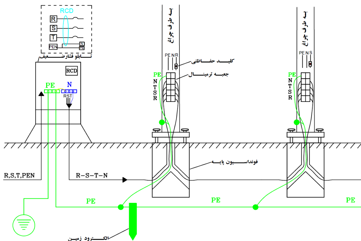
شکل ۶-۴- سیستم توزیع زمین TN-C-S در تغذیه چراغ‌های روشنایی معابر و نحوه اتصال کلید RCD
