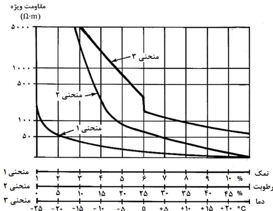
شکل ۱-۳- تاثیر میزان رطوبت، دما و نمک بر مقاومت ویژه [۲]
